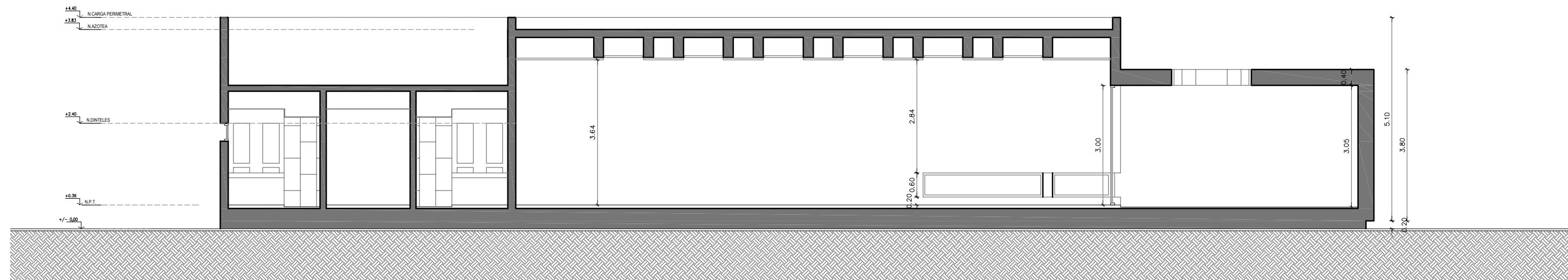
ARQUITECTURA - CORTE LONGITUDINAL C-C
